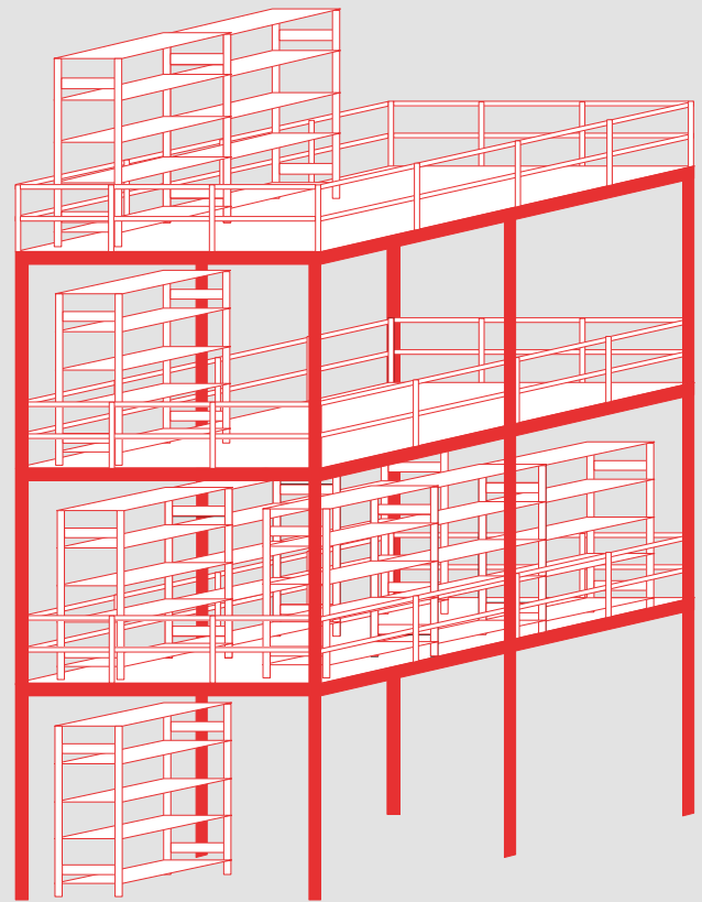
4 -geschossige Bühnenanlage → 12 Meter Regalhöhe möglich
