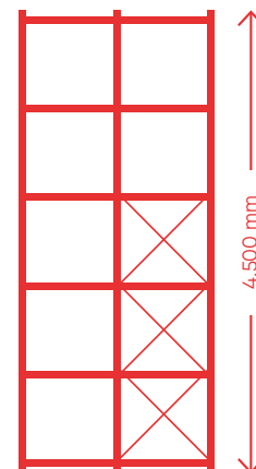
bis H = 4.500 mm: 3 Kreuzstreben
